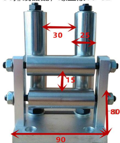
30排线器配，螺丝眼60*62
