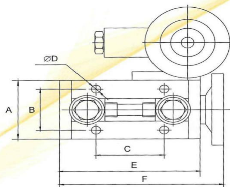
TX25-110四辊可调导线装置技术参数表
