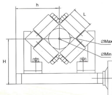
TX25-110斜辊可调导线装置技术参数表
