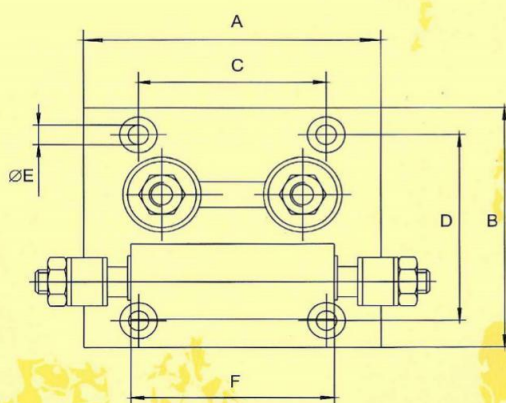
TX30-50井字型导线装置技术参数表
